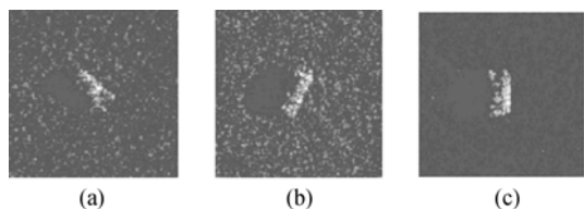
图2 在不同方位角下的 SAR 原始目标图像 (a) BMP2, 320^\circ ; (b) BTR70, 62^\circ ; (c) T72, 90^\circ
