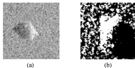
图4 (a)和(b)分别是目标 T72 预处理前后的 SAR 图像
