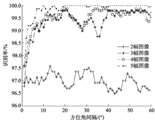
图7 多方位角图像决策融合的识别率
