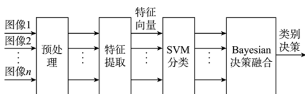
图1 SAR 图像目标识别过程框图
