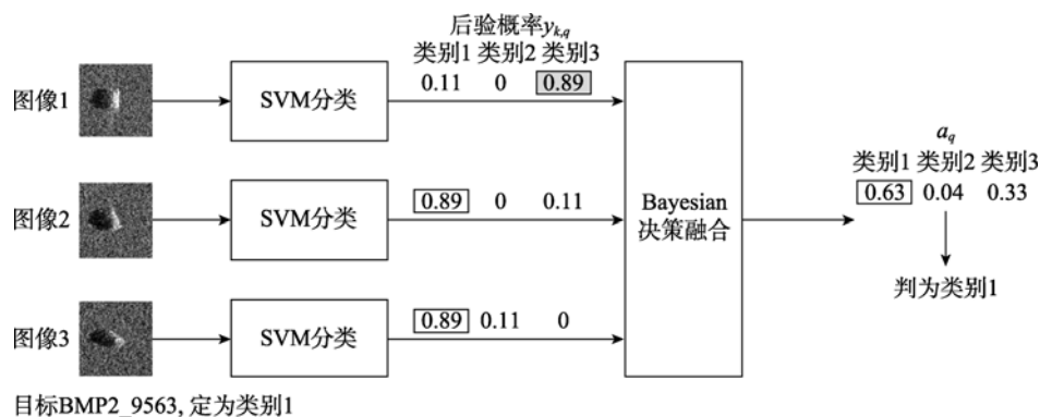
图6 贝叶斯决策融合过程示意图
